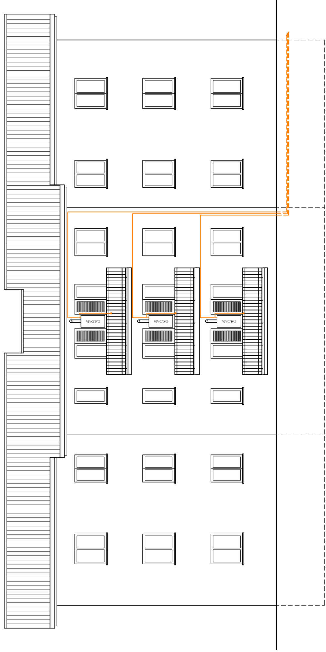
Prospetto Posteriore scala 1:100
