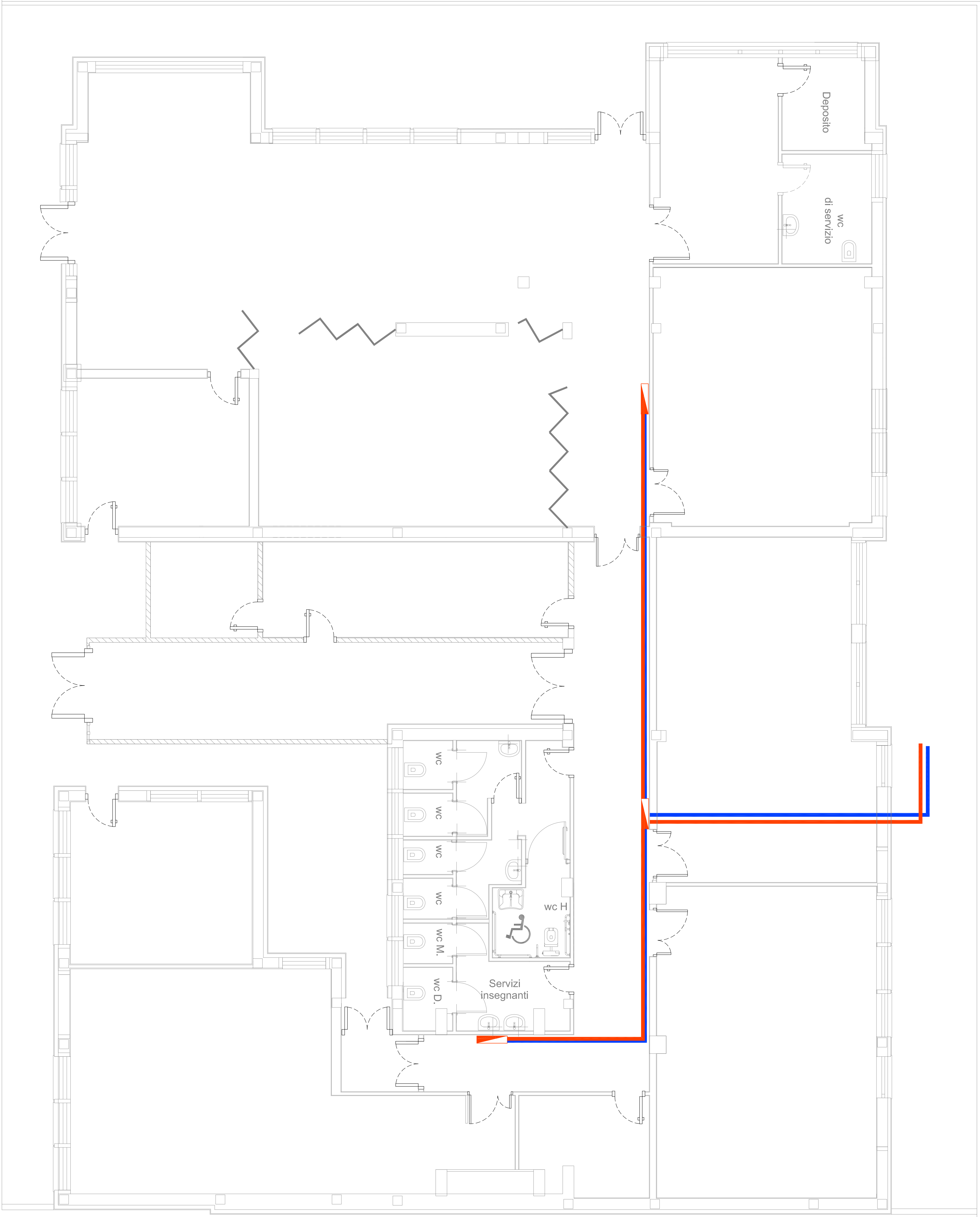
PIANTA DORSALI IMPIANTO TERMICO - Scala 1:50
