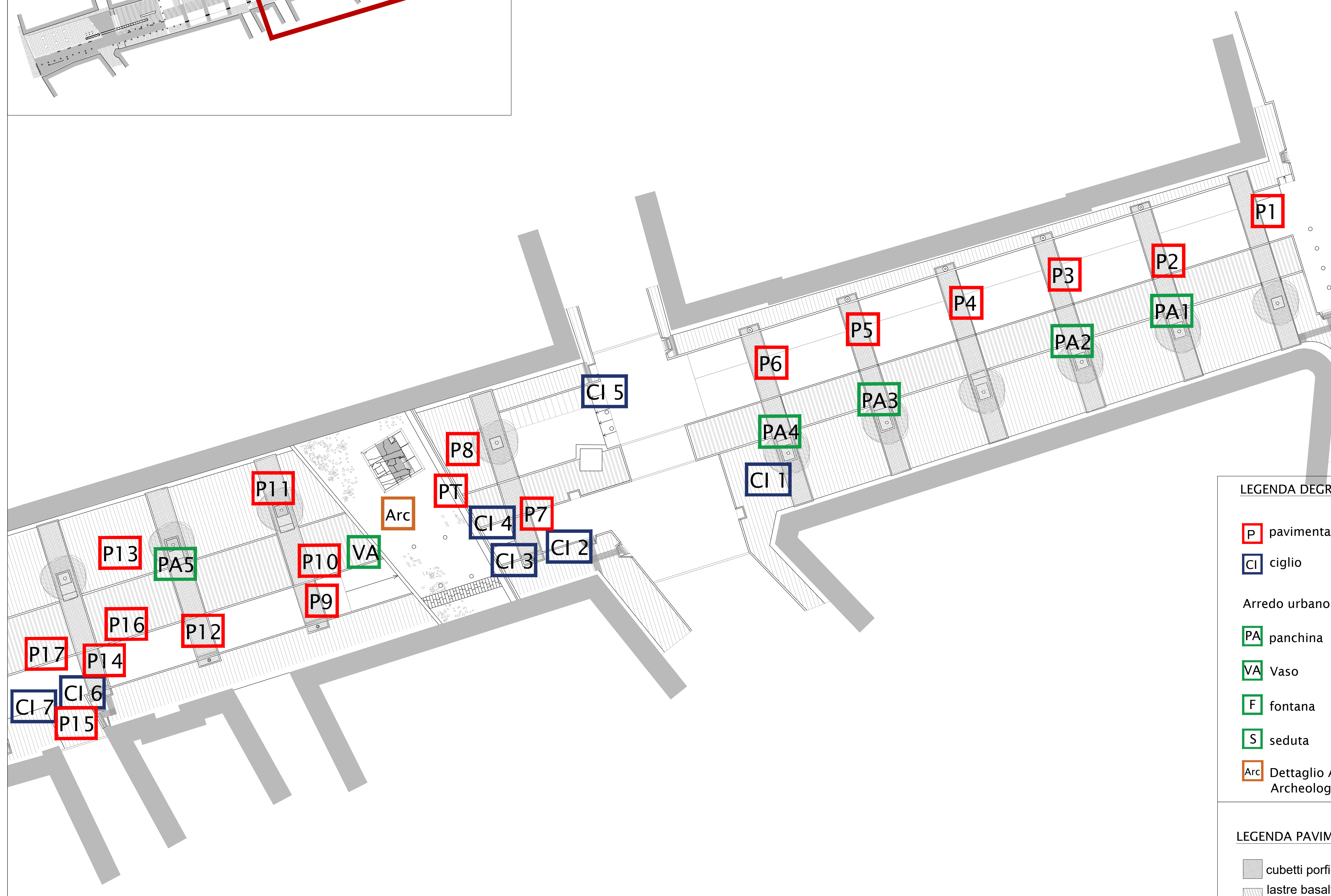
planimetria | scala 1:200
