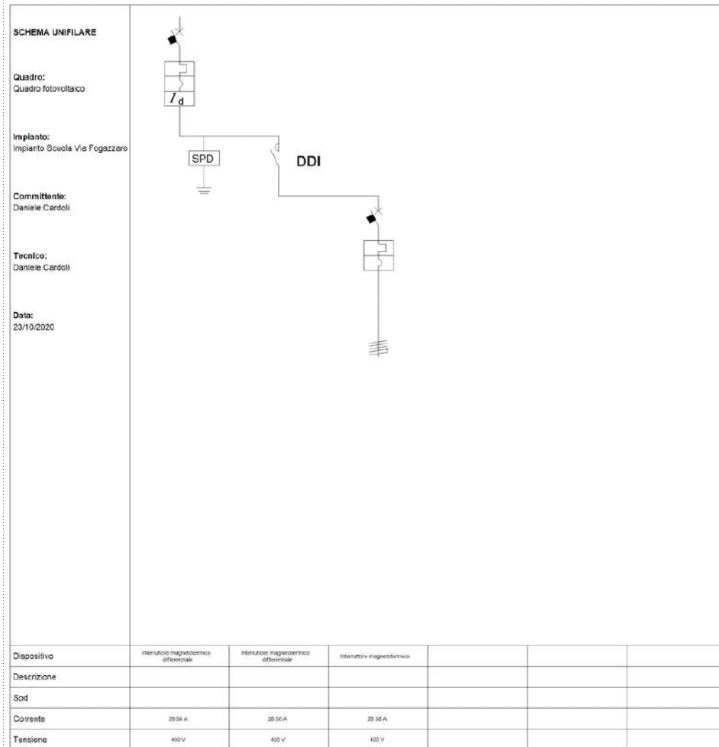
Fig. 7: Schema unifilare quadro "Quadro fotovoltaico"
