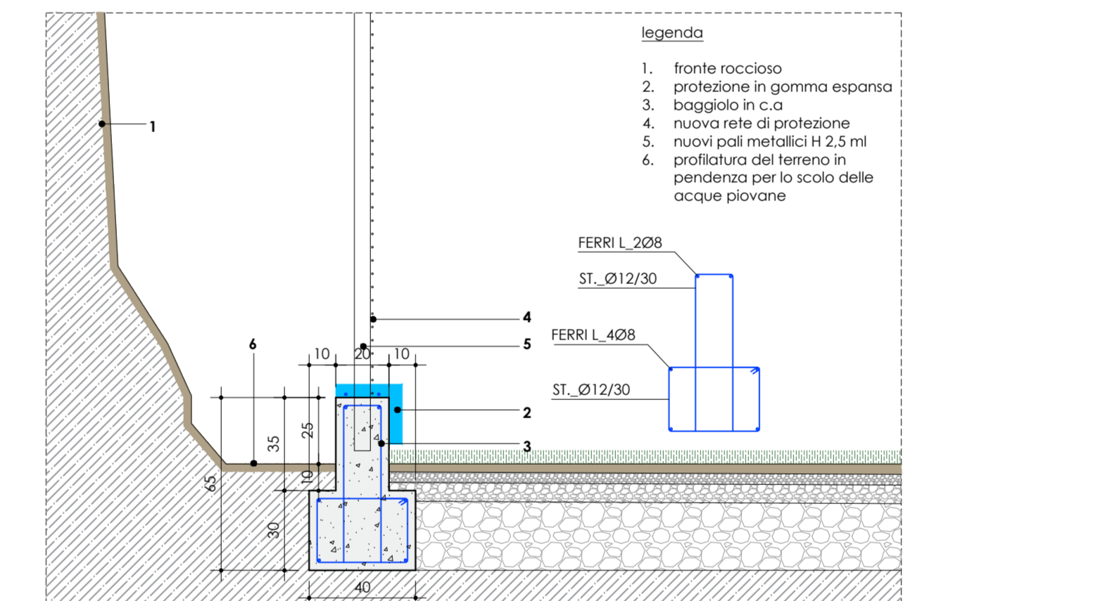
Particolare costruttivo baggiolo scala 1:20
