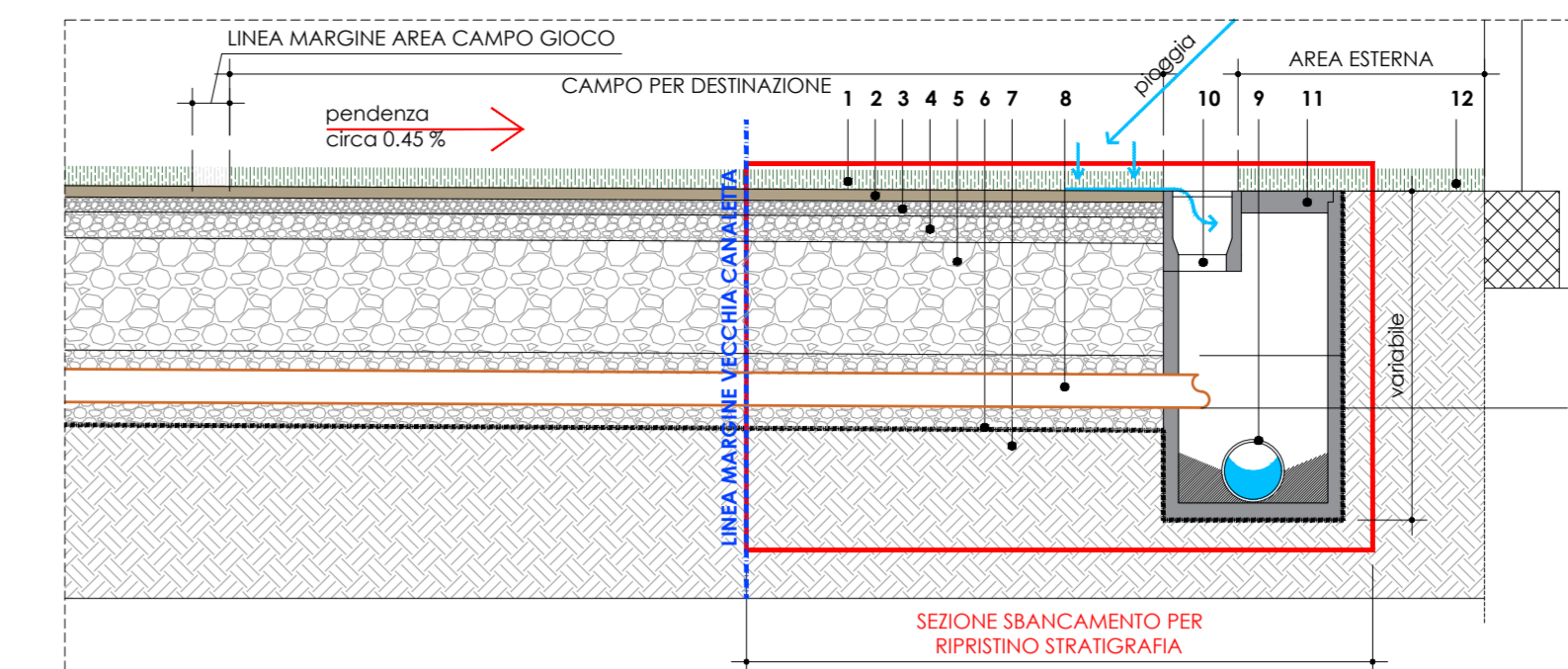
Particolare costruttivo drenaggio perimetrale scala 1:20
