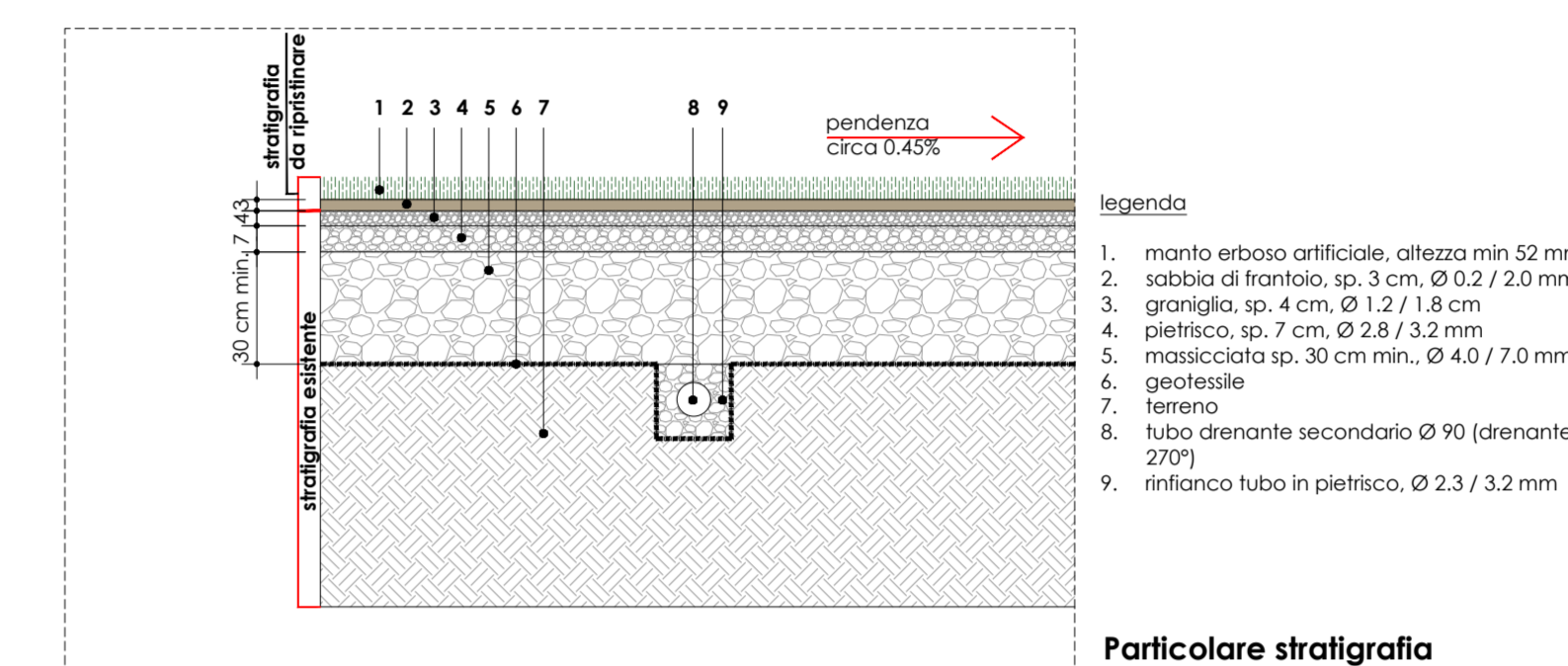
Particolare stratigrafia scala 1:20
