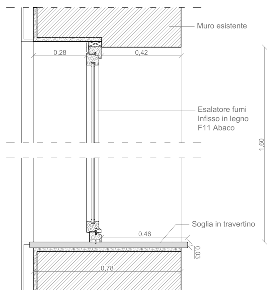
SD16_ SEZIONE DETTAGLIO INFISSO PIANO SECONDO_SCALA 1: 10
