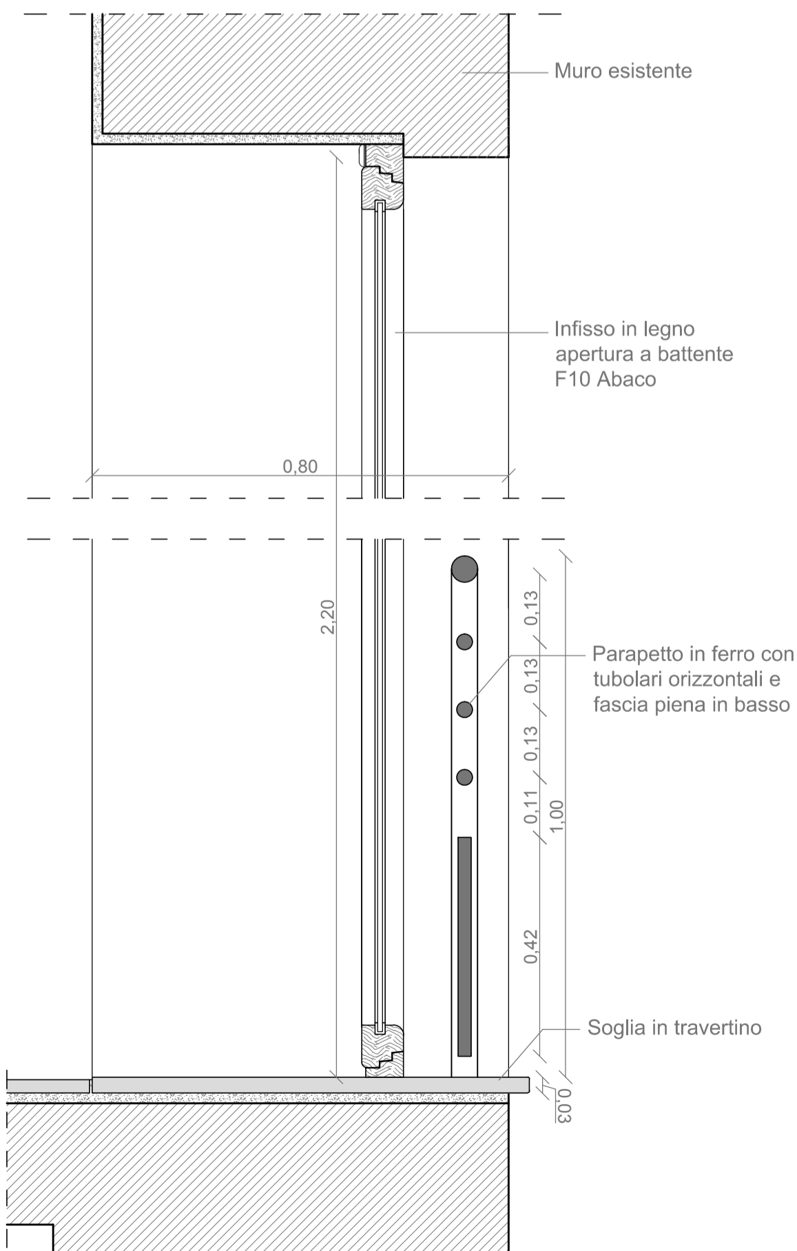
SD15_ SEZIONE DETTAGLIO INFISSO PIANO -1 E SECONDO_SCALA 1: 10
