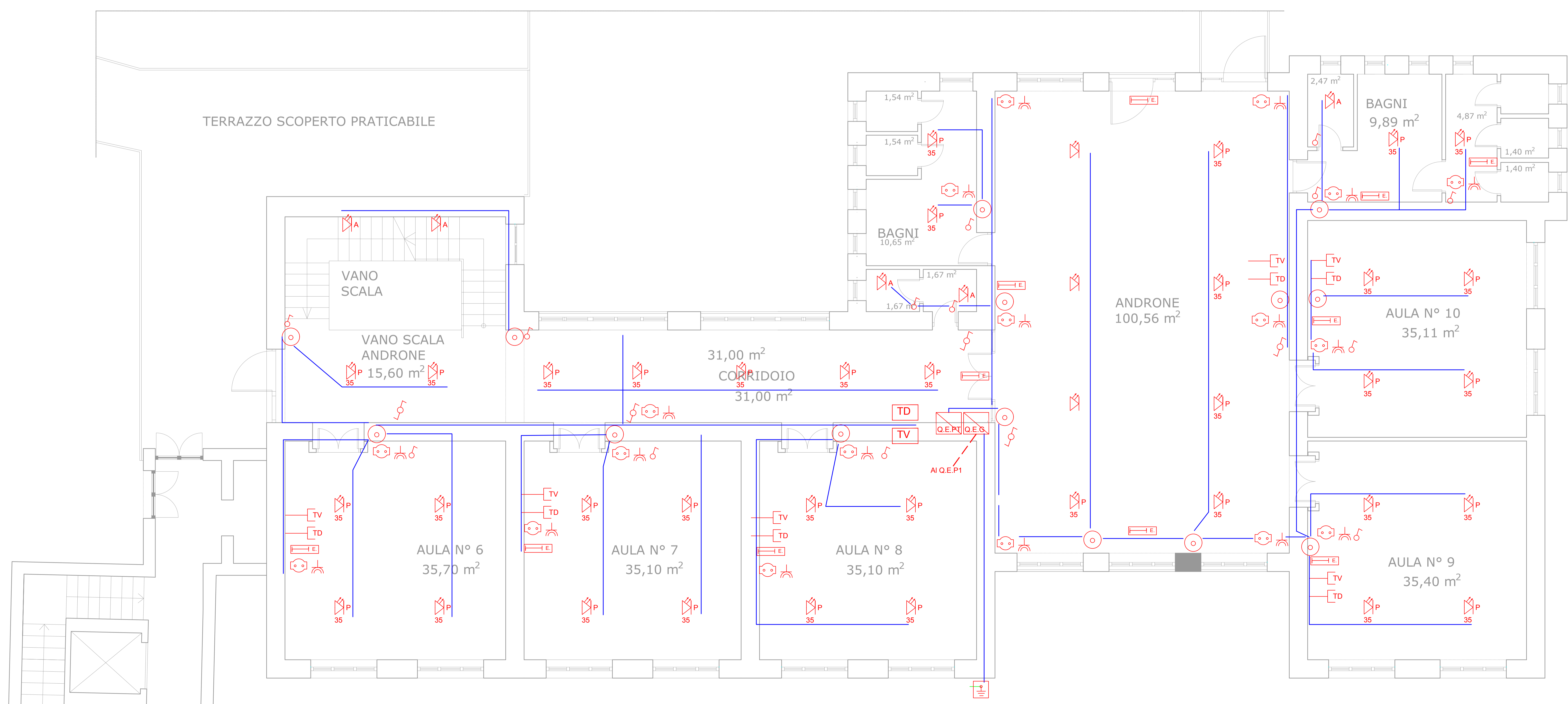
Schema planimetrico unifilare con disposizione topografica dei componenti
